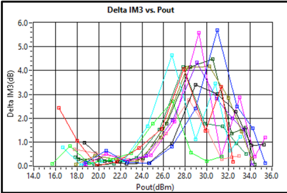
Delta IM 3 vs. Output Power 19GHz – 39GHz
