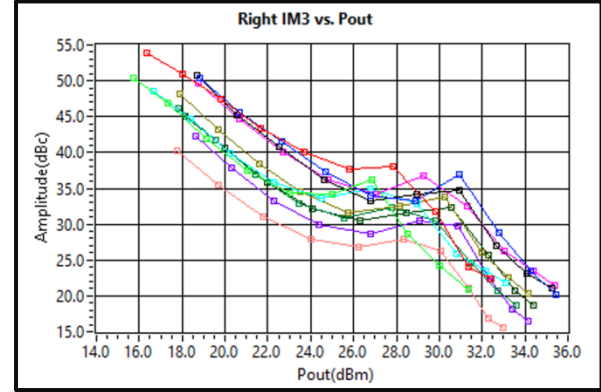
Right IM 3 vs. Output Power 19GHz – 39GHz
