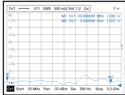
Input VSWR@+25°C
