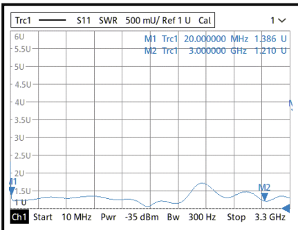
Input VSWR@-40°C
