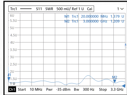
Input VSWR@+70°C
