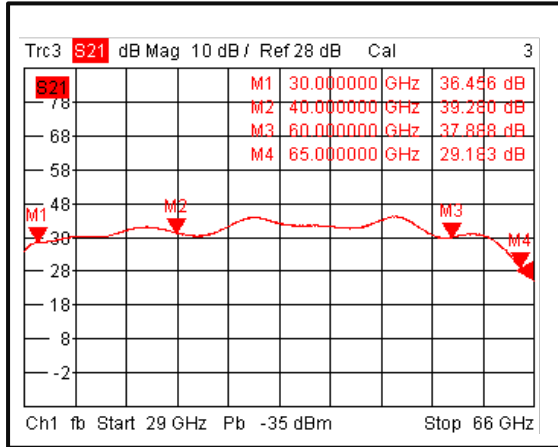
Output VSWR@-45°C
