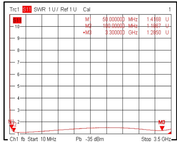
Input VSWR@+85°C
